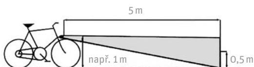
Centrování předního reflektoru
